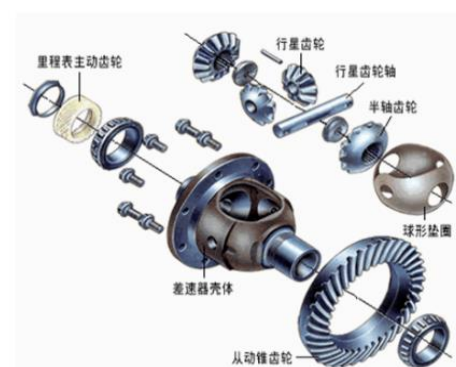
传统汽车差速器总成结构图
